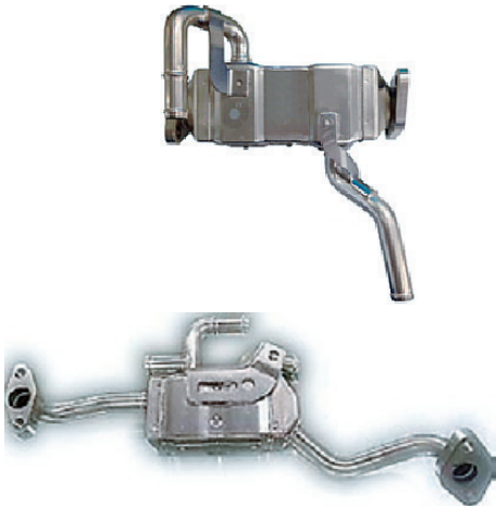
乗用車クラス向EGRクーラー
